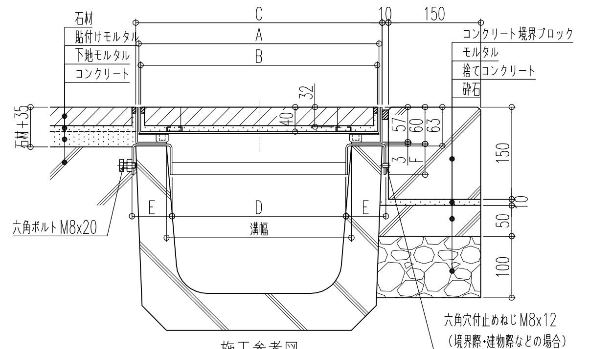
施工参考図
